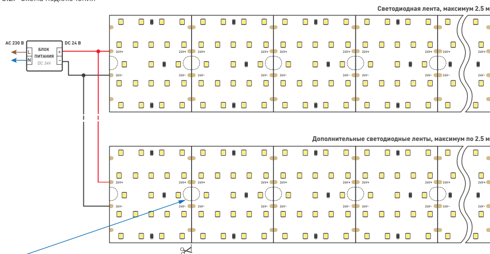
Схема 1. Подключение нескольких светодиодных лент
