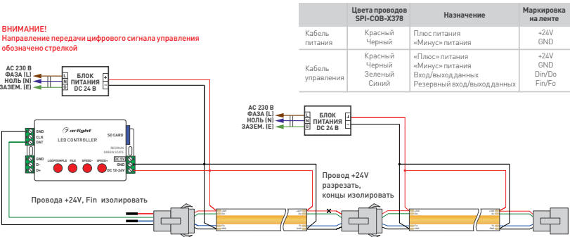
Схема 1. Схема подключения ленты с использованием SPI-контроллера с одним выходным портом и с использованием отдельных блоков питания
