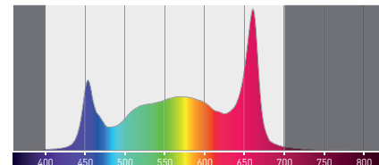
Данный спектр излучения представлен для ленты FITOLUX-A66-8mm 24V
