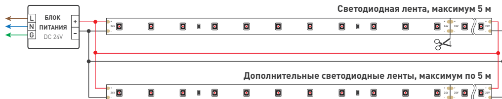
Схема 1. Подключение нескольких светодиодных лент с двух сторон
