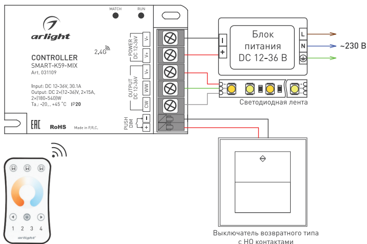
Рисунок 1. Схема подключения контроллера SMART-K59-MIX
